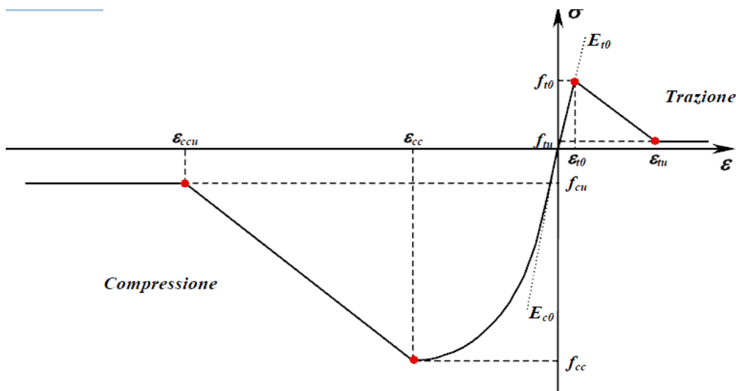
Figura 2.14: curva analitica uniaxiale deformazioni-sforzi ( \varepsilon - \sigma ) per il c.a.
