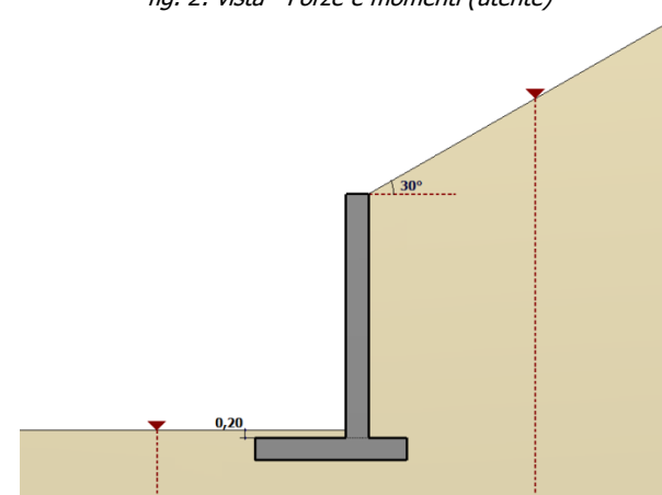
fig. 4: profilo Terreno
