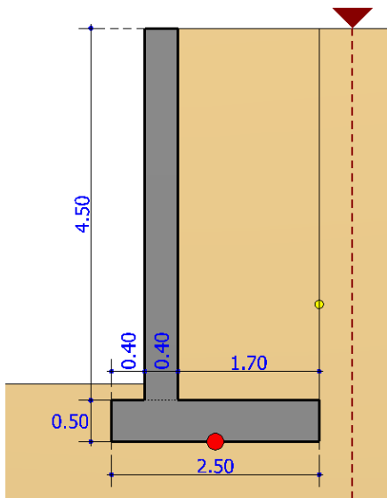
fig. 1. Punto di rotazione e Geometria Muro
