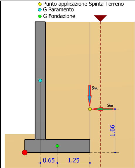
fig. 3. Dati Pesi muro e Spinte terreno (orizzontale e verticale)
