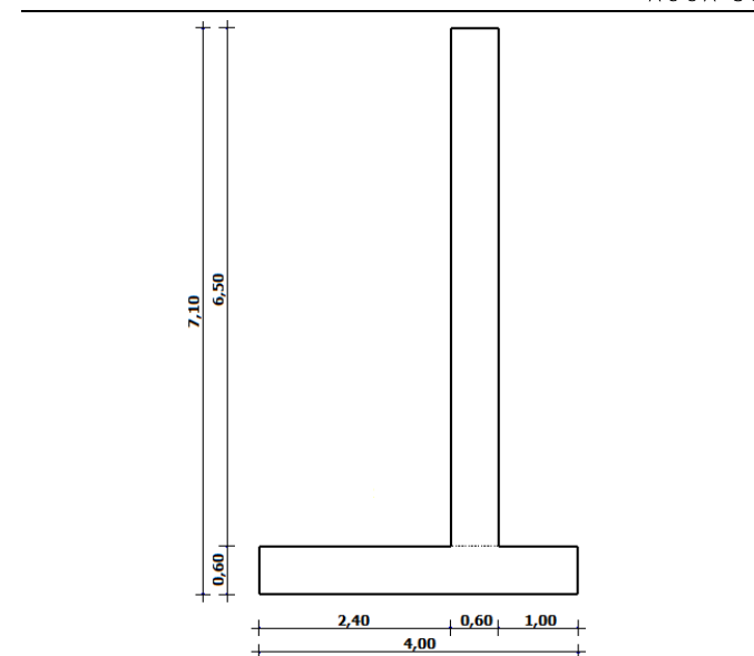
fig. 1: geometria Muro
