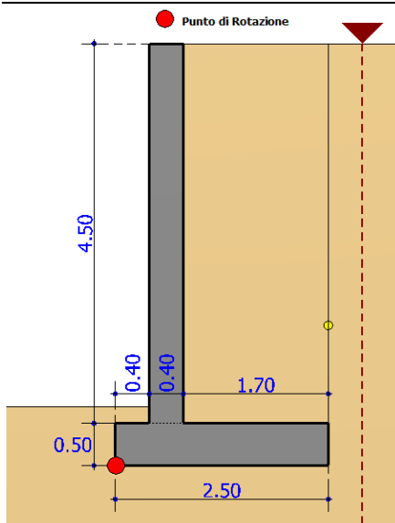
fig. 1. Punto di rotazione e Geometria Muro
