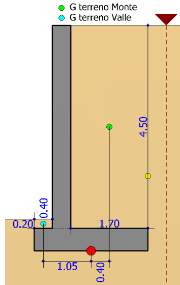
fig. 2. Dati terreno a Monte/Valle
