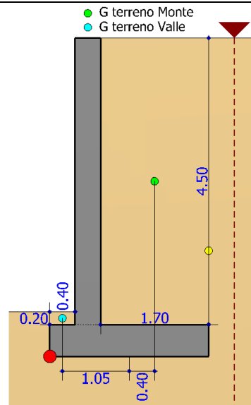
fig. 2. Dati terreno a Monte/Valle
