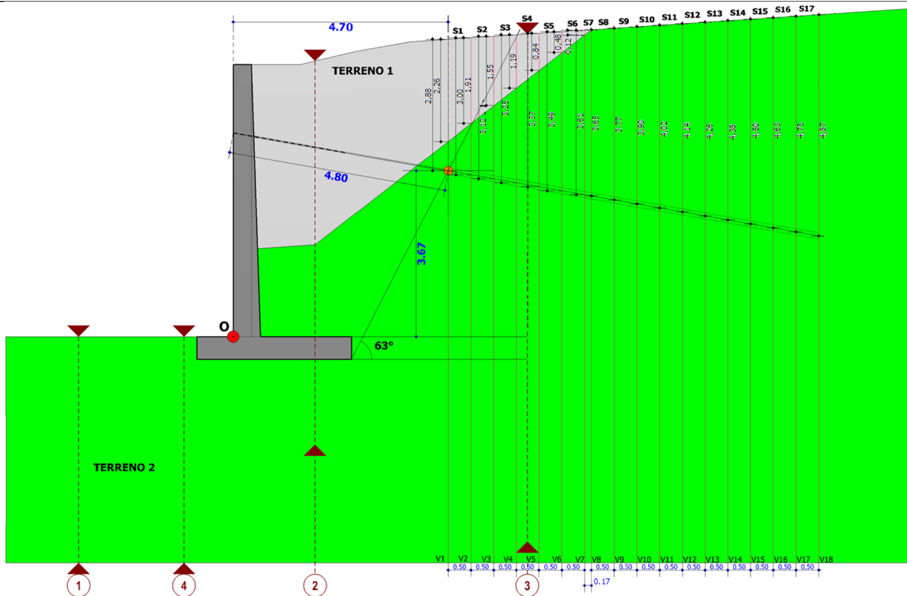
fig. 7: Discretizzazione del volume di terreno (verticali e settori/strisce) dell'iterazione finale
