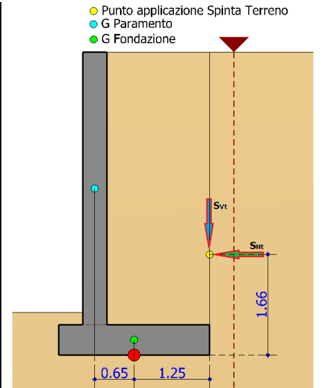
fig. 3. Dati Pesì muro e Spinte terreno (orizzontale e verticale)
