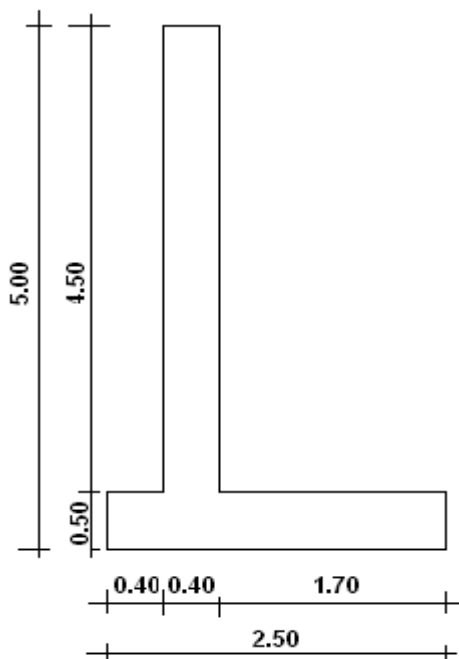
fig. 1. Geometria Muro
