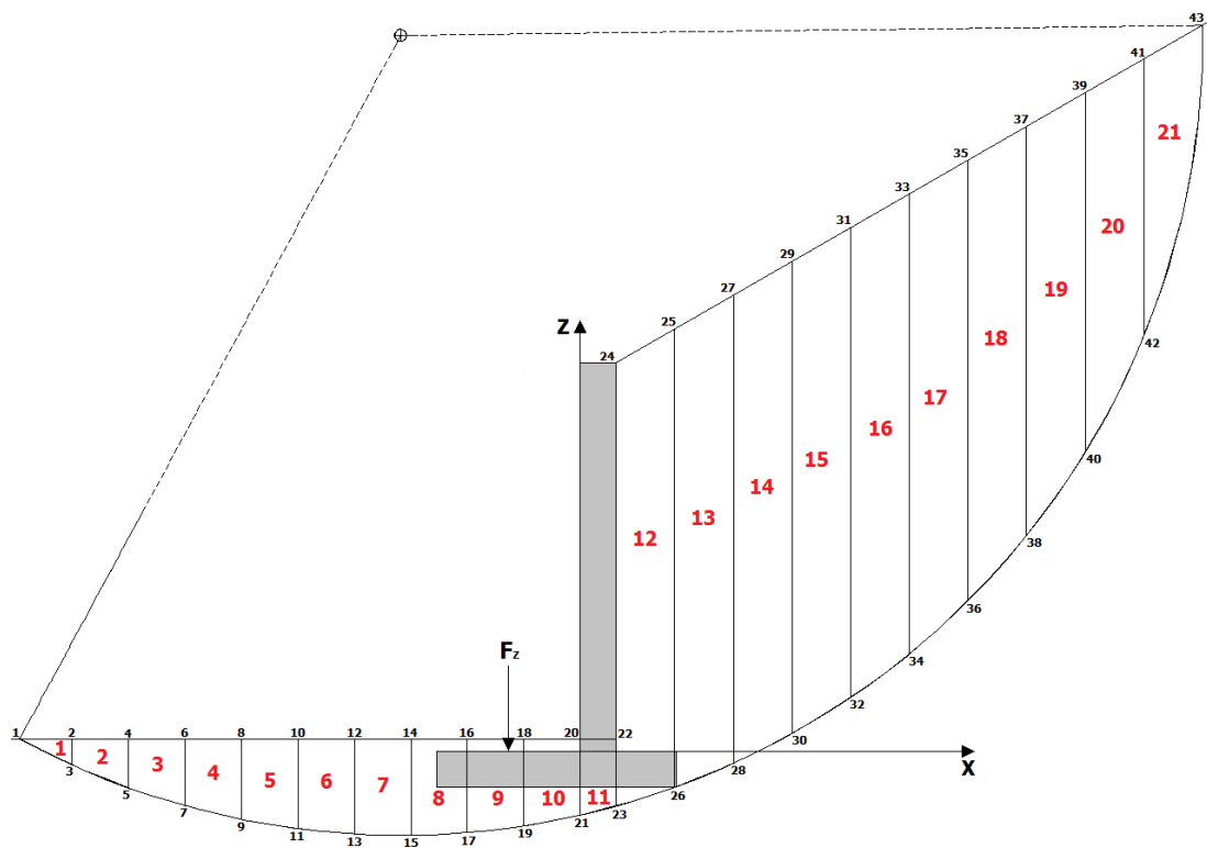
fig. 6: individuazione strisce
