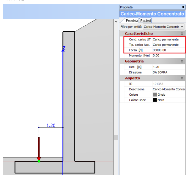
fig. 2: vista - Forze e momenti (utente)
