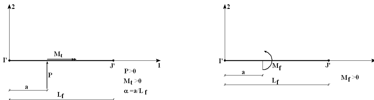
Figura 2.10: carichi concentrati
