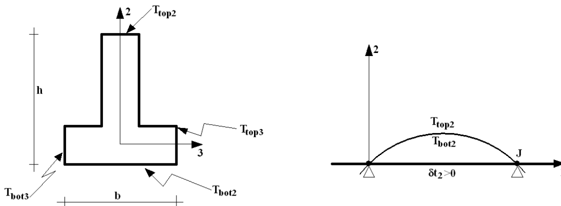
Figura 2.9: gradiente termico
