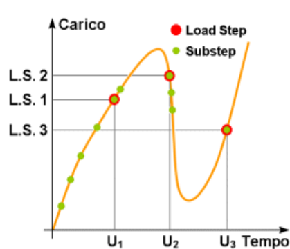
Figura 4.2: soluzione nella curva carichi spostamenti
