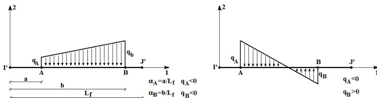
Figura 2.11: carichi ripartiti
