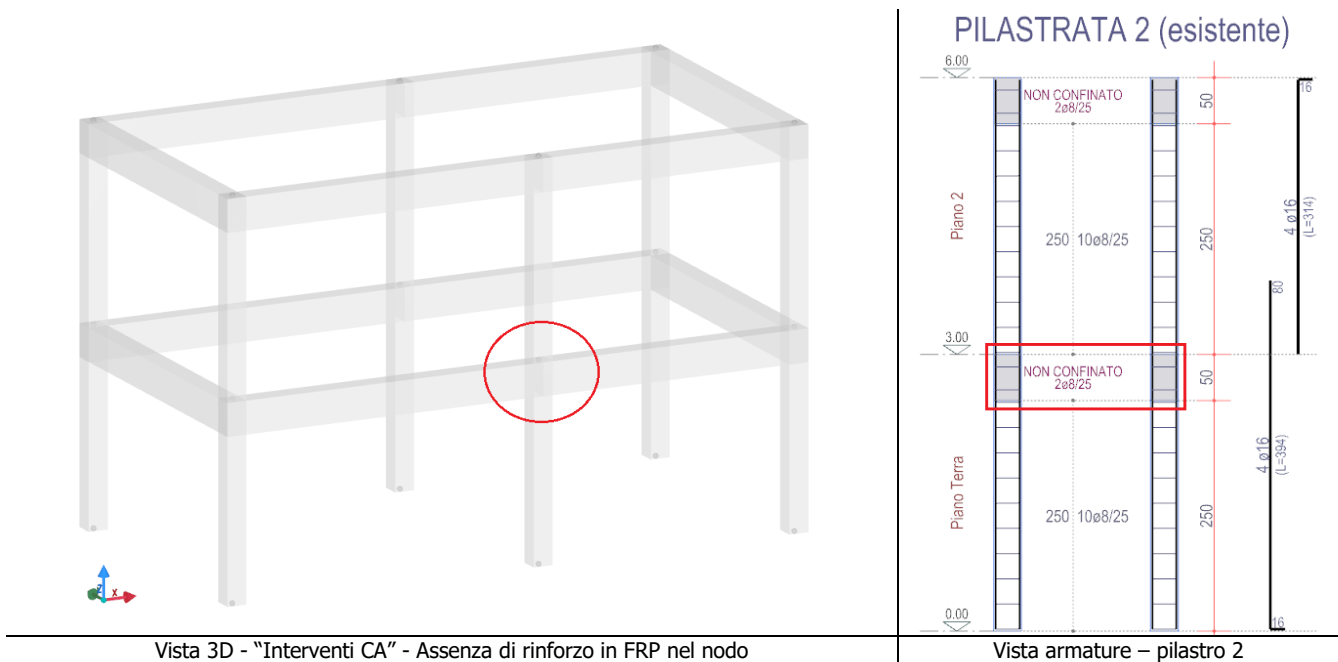
Figura 10.6: nodo con staffe nel nodo ma senza rinforzo in FRP
