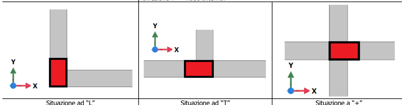
Figura 10.3: posizione nodo - Interno/Esterno
