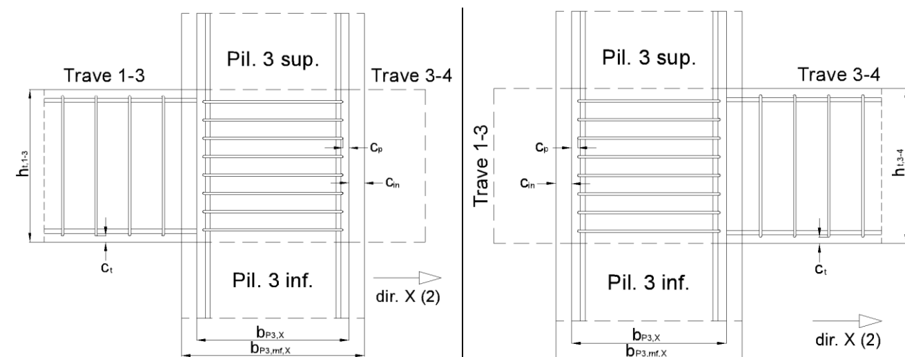
Figura 15.4: viste/sezioni in pianta e prospettive delle travi che entrano/escono dal nodo - direzione X
