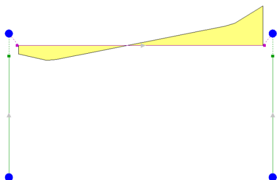
Figura 14.5: momento flettente ( M_3 ) per sisma "+X - proporzionale alla deformata 1° modo di vibrazione"
