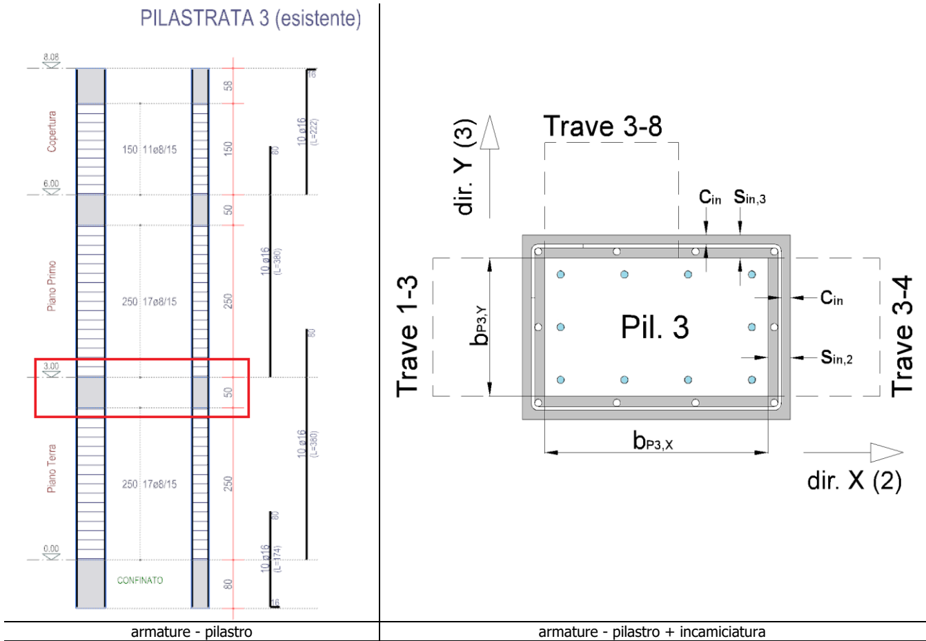
Figura 15.3: armature - pilastro
