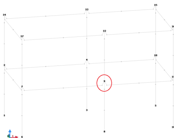
Figura 10.2: vista - "Strutturale"
