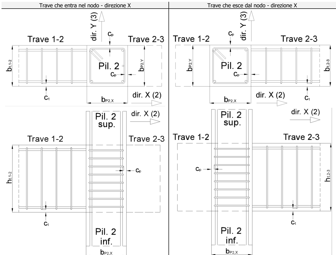
Figura 10.4: viste/sezioni in pianta e prospetto delle travi che entrano/escono dal nodo - direzione X
