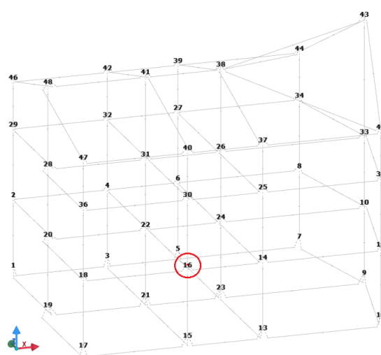
Figura 15.2: vista - "Strutturale"
