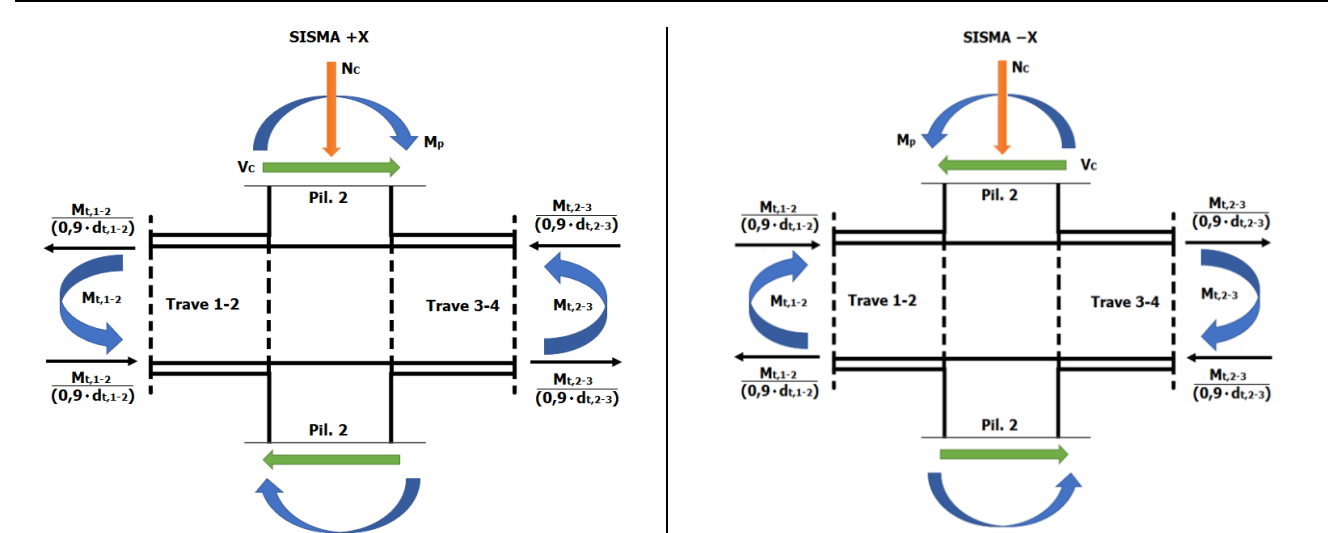
Figura 15.7: azioni agenti sul nodo per sisma +/-
