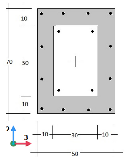
Figura 7.6: sezione rinforzata
