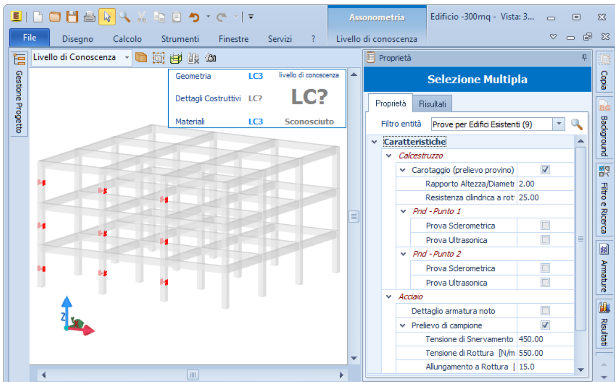
Figura 1.12: LC3 - Materiali
