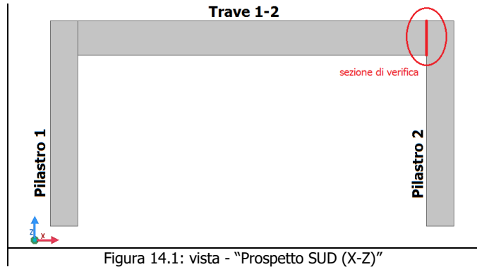
Figura 14.1: vista - "Prospetto SUD (X-Z)"
