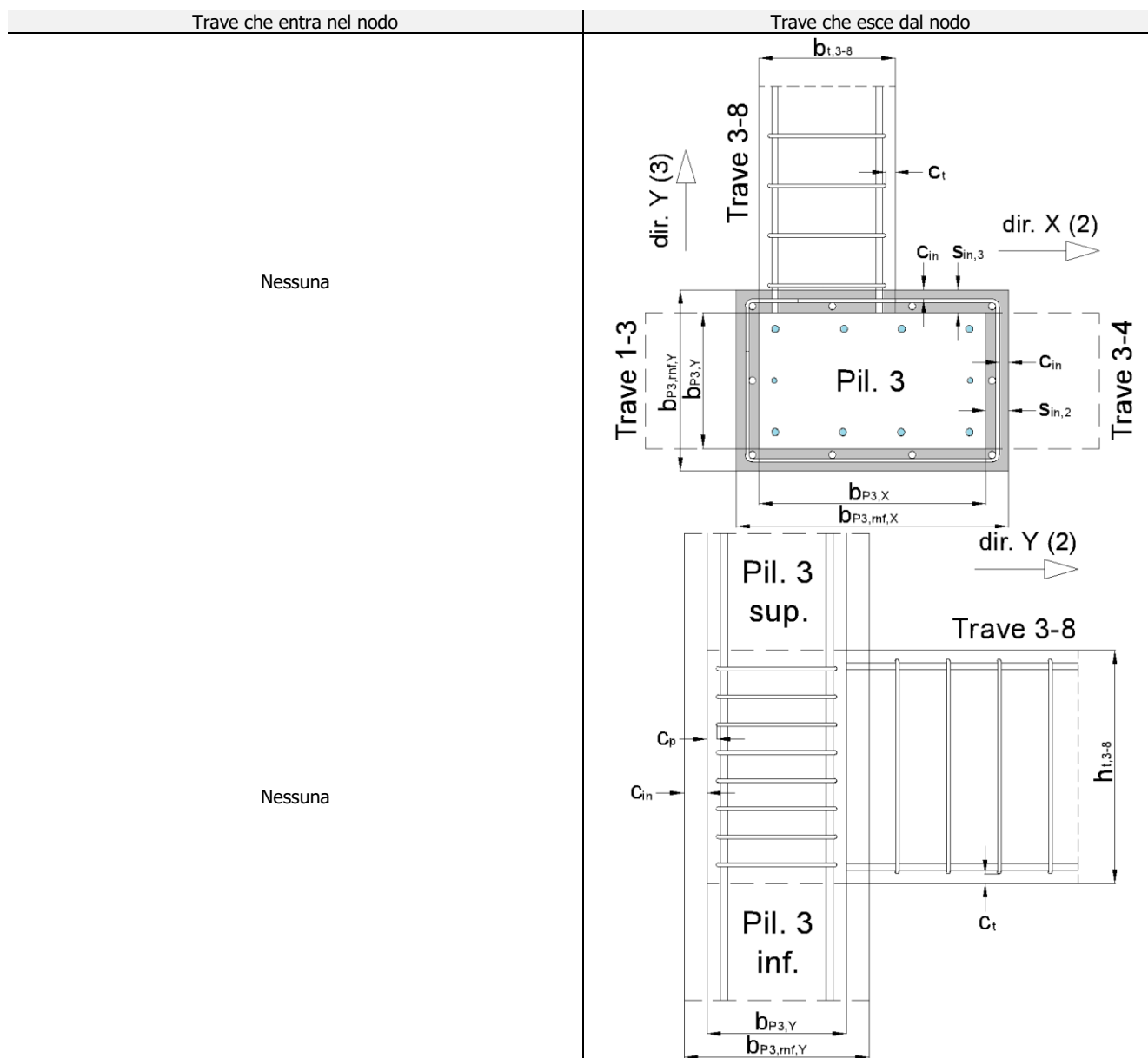
Figura 15.5: viste/sezioni in pianta e prospetto delle travi che entrano/escono dal nodo - direzione Y
