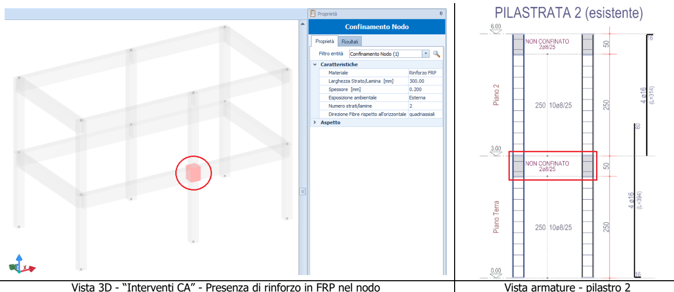
Figura 10.7: nodo con staffe + rinforzo in FRP
